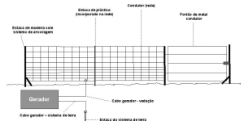
Componentes de uma vedação eléctrica móvel de rede
