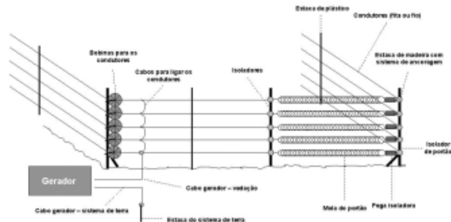
Componentes de uma vedação eléctrica móvel de fios ou fitas
